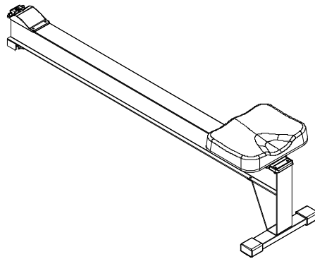
NO:50
