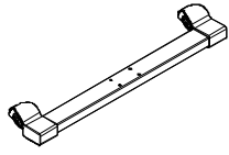
NO:55
